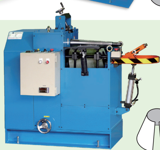
CMRS 油壓錐度捲圓機 特殊型 Hydraulic Taper Rolling Machine (special type)
