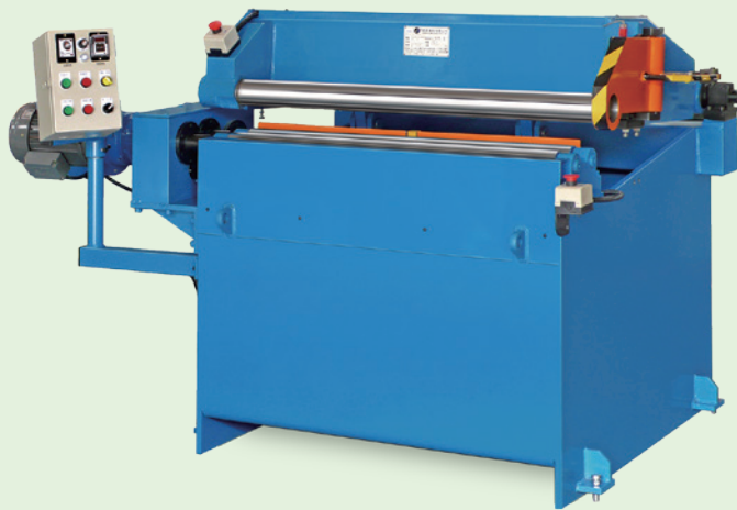
CMRD 油壓三軸捲圓機 特殊型 Hydraulic 3-shaft Rolling Machine (special type)
