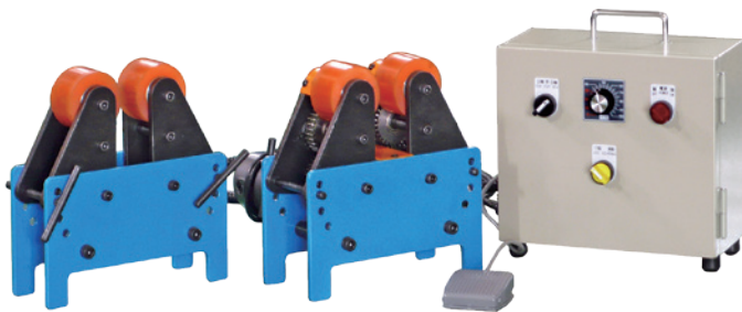
CMSA-500K Max. load 最大荷重: 0.5T
